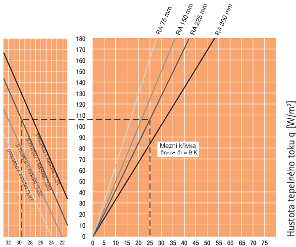
Teplota povrchu podlahy t (°C) Využitelný rozdíl teplot \Delta\theta_H [K]
