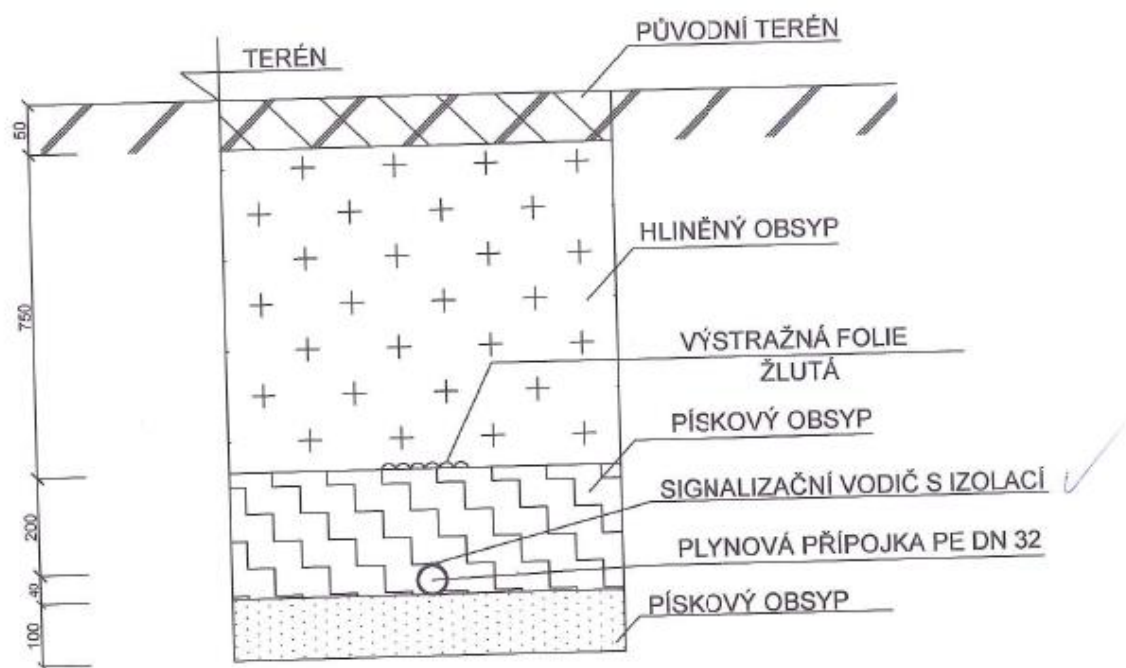
PŘÍČNÝ ŘEZ RÝHY PŘI UKLÁDÁNÍ DOMOVNÍ PŘÍPOJKY
