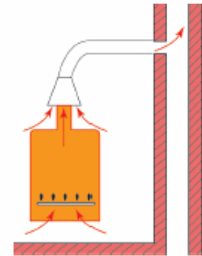
Schéma spotřebiče typu B
