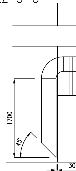
ŘEZ C-C
