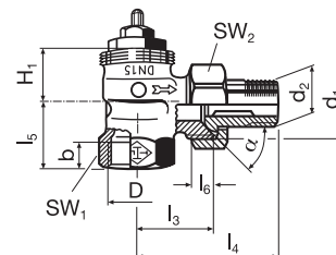
Radiátorové ventily rohové (ET) se zkrácenými stavebními rozměry 2215; 3505; 3515
