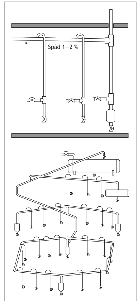
Obr. 2.22. Příklad na vytvoření potrubní sítě
