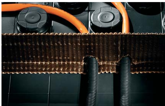
4b. Deska přívodu s dilatačním pásem 1 m
