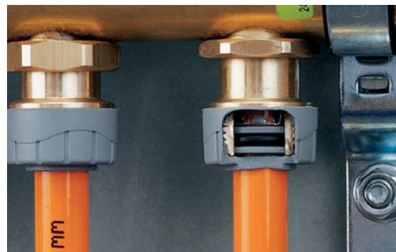
7. Řez hotovým násuvným spojem
