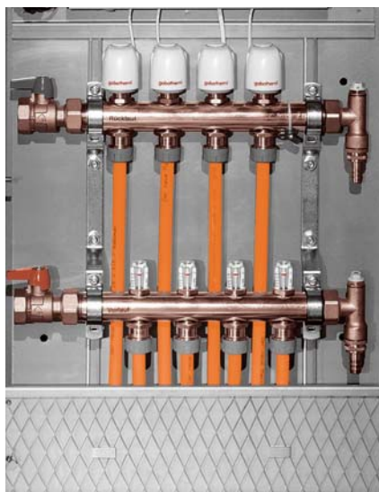
5. Detail připojení trubek k rozdělovací stanici
