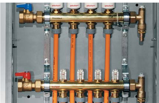
8. 1.2.3 – a montáž je hotová!
