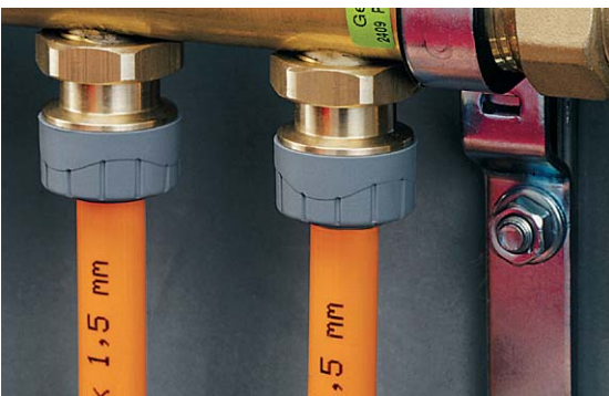
6e. Konec trubky se zasune do násuvné spojky
