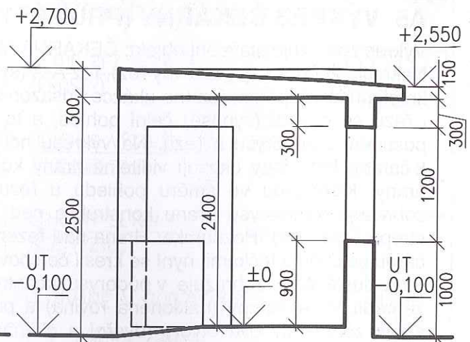
ŘEZ A-A
